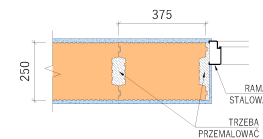
- WIĄZANIE PRZY OKŁADZINIE DRZWI, 1. RZĄD MURÓW
