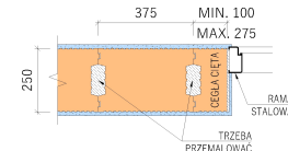
- WIĄZANIE PRZY OKŁADZINIE DRZWI, 2. RZĄD MURÓW
