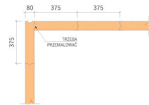
- WIĄZANIE NAROŻNE, 2. RZĄD MURÓW
