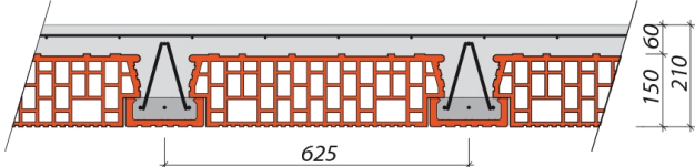
Grubość stropu 210 mm - maks. długość belki stropowej 6 250 mm
