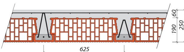
Grubość stropu 250 mm
