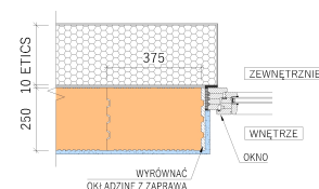
- WIĄZANIE PRZY OKŁADZINIE OKIENNEJ, 1. RZĄD MURÓW
