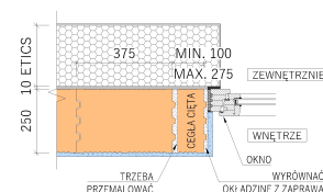
- WIĄZANIE PRZY OKŁADZINIE OKIENNEJ, 2. RZĄD MURÓW
